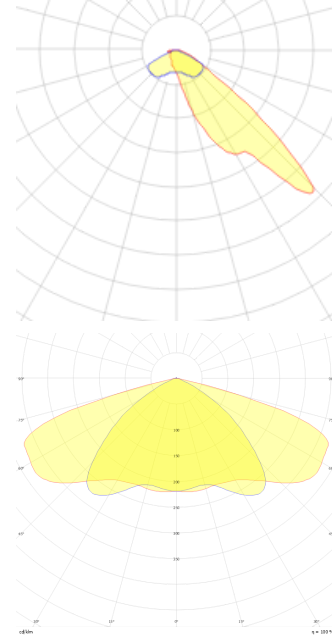
Fotometrik Eğri
