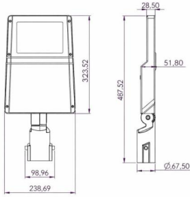
Teknik Çizim
