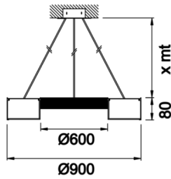
Teknik Çizim
