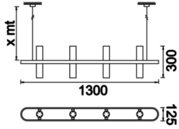
Teknik Çizim
