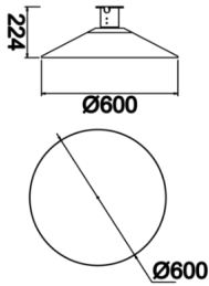
Teknik Çizim
