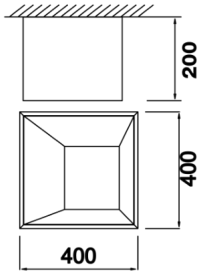
Teknik Çizim
