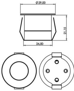
Teknik Çizim
