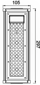
Teknik Çizim
