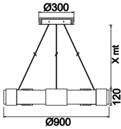
Teknik Çizim
