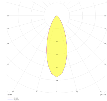
Fotometrik Eğri
