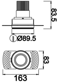
Teknik Çizim
